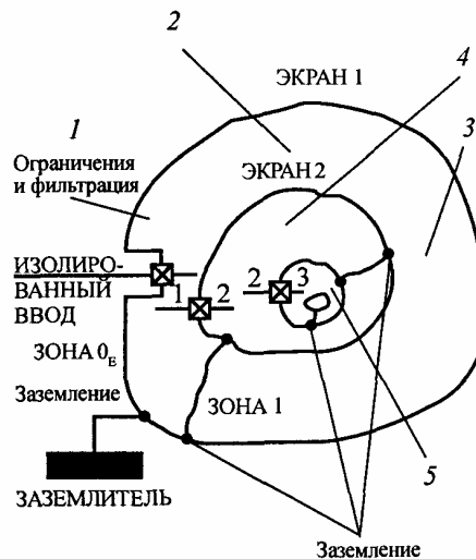
Рис. 4.1. Зоны защиты от воздействия молнии: 1 - ЗОНА 0 (внешнее окружение); 2 - ЗОНА 1 (внутренняя электромагнитная обстановка); 3 - ЗОНА 2; 4 - ЗОНА 2 (обстановка внутри шкафа); 5 - ЗОНА 3
