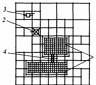
Рис. 4.8. Сетчатое заземляющее устройство производственных сооружений: 1 - здания; 2 - башня; 3 - оборудование; 4 - кабельный лоток
