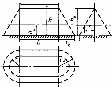
Рис. 3.2. Зона защиты одиночного тросового молниеотвода:
