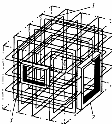
Рис. 4.3. Объединение металлических элементов объекта для уменьшения влияния электромагнитных полей: 1 - сварка на пересечениях проводов; 2 - массивная непрерывная дверная рама; 3 - сварка на каждом стержне
