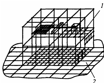
Рис. 4.7. Сетчатое заземляющее устройство здания: 1 - сеть соединений; 2 - заземлитель
